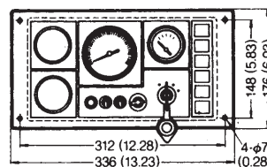
Type C (4JH3-DTE)
